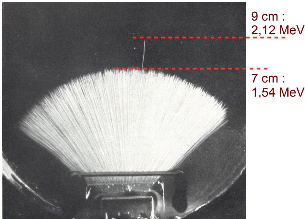
Nebelkammer-Spuren von \alpha -Teilchen
