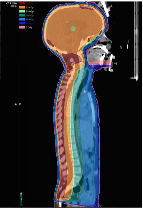
Röntgenstrahlen
