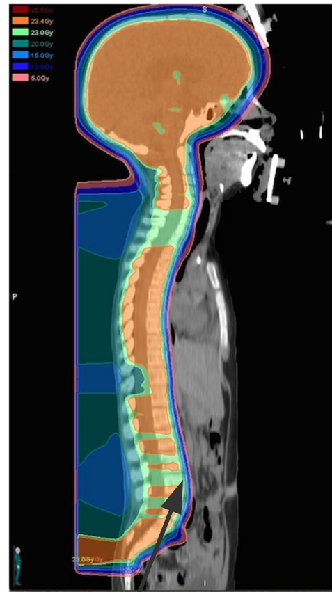
Schwere Ionen
