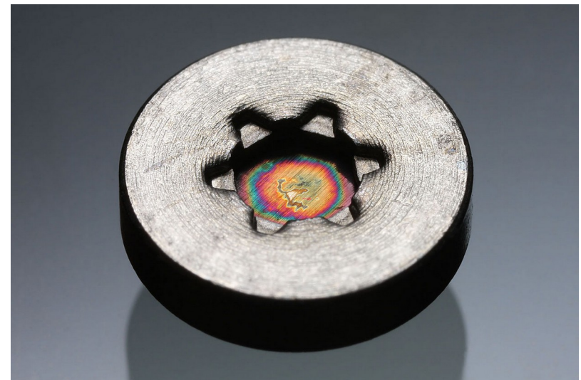
^{241}\text{Am} -Quelle aus einem Ionisations-Rauchmelder.
